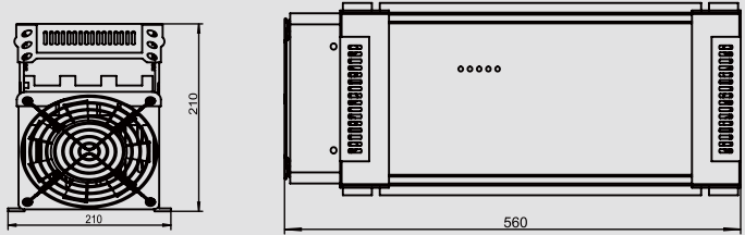
GSM3K40600D 长宽高:560mm*210mm*210mm
