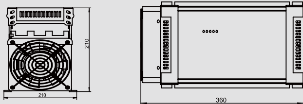
GSM3K40400D 长宽高:360mm*210mm*210mm
