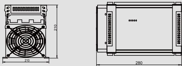
GSM3K40250D-SAM3K40300D 长宽高:280mm*210mm*210mm
